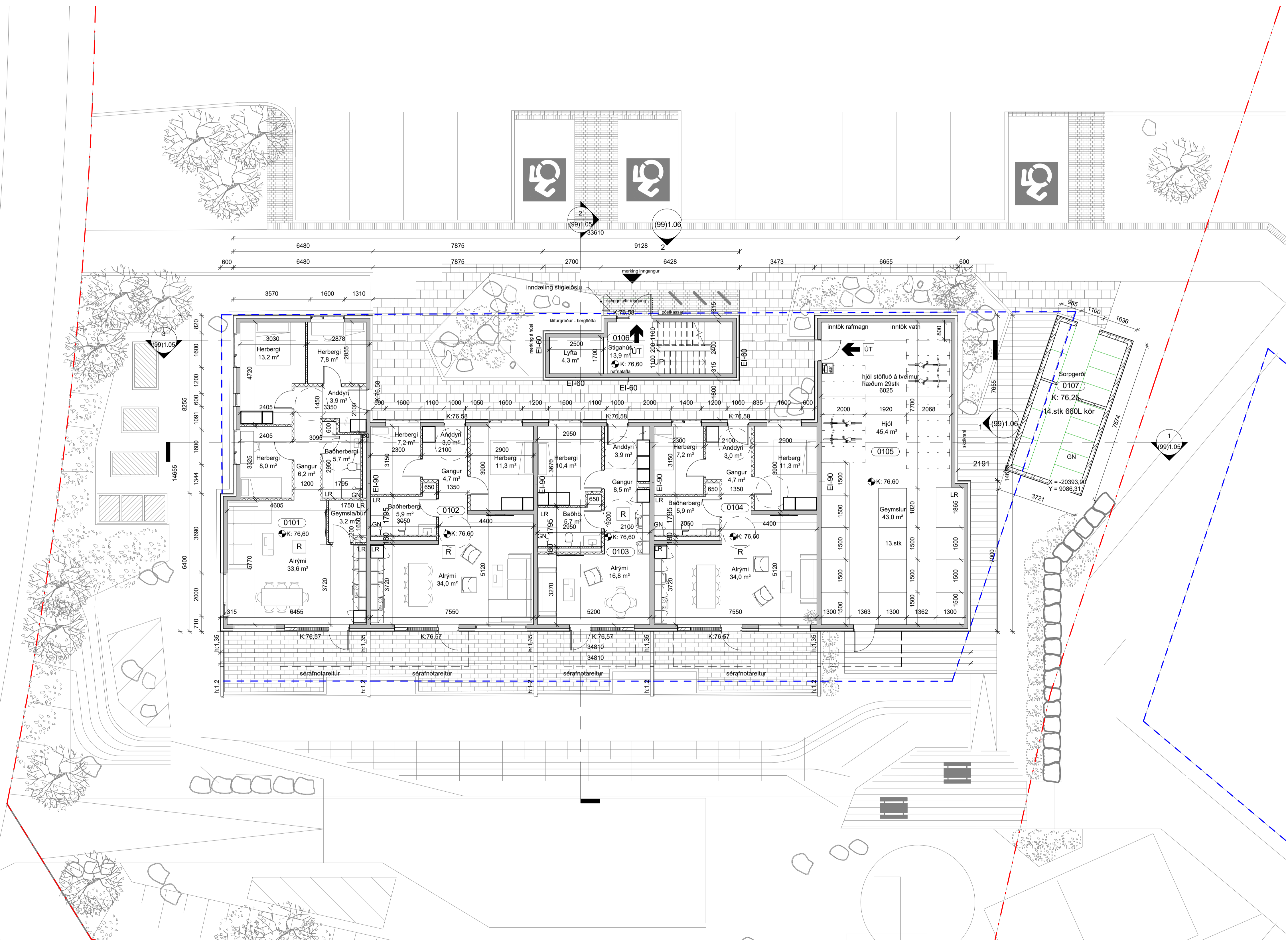
1 Grunnmynd, 1. hæð 1 : 100
