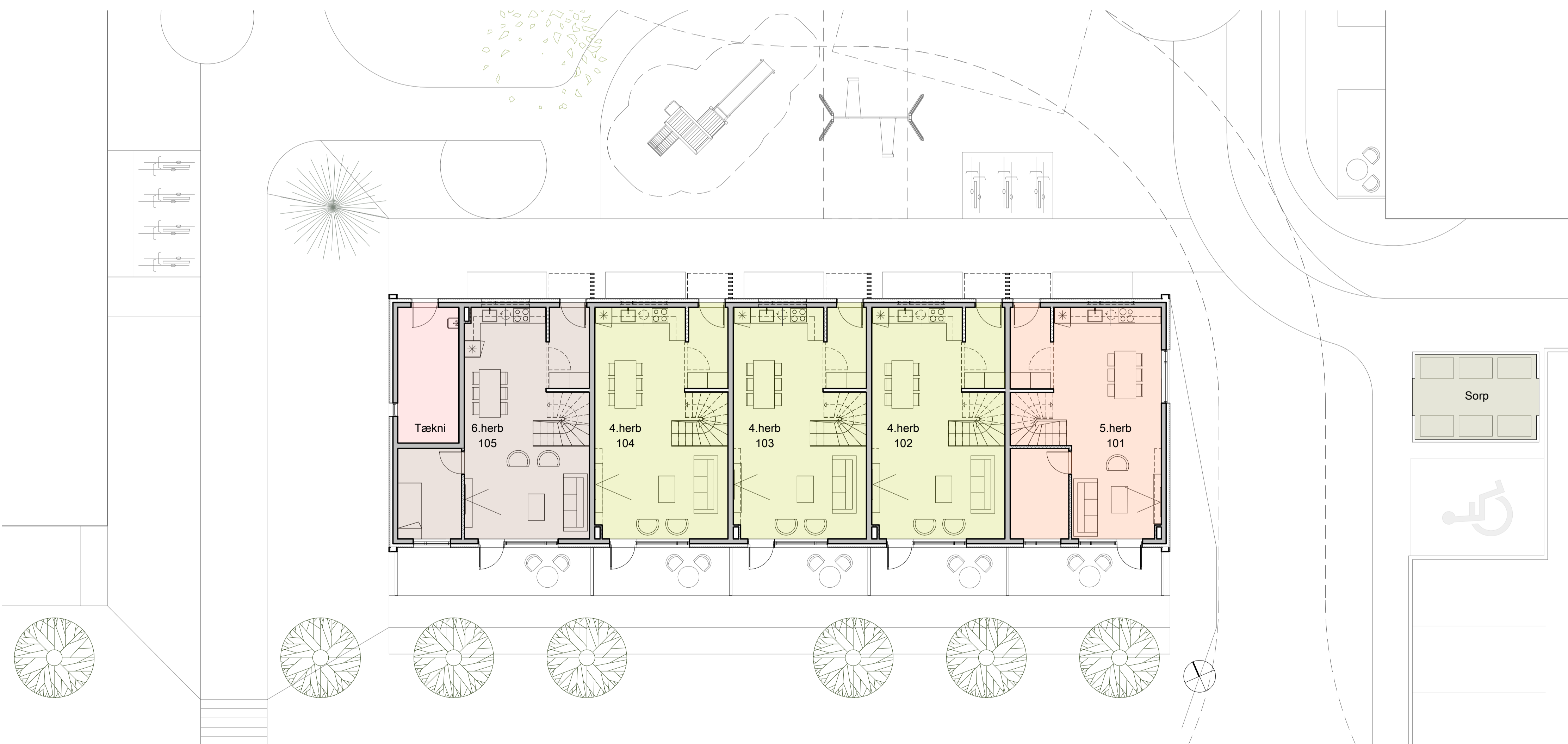
1.hæð
