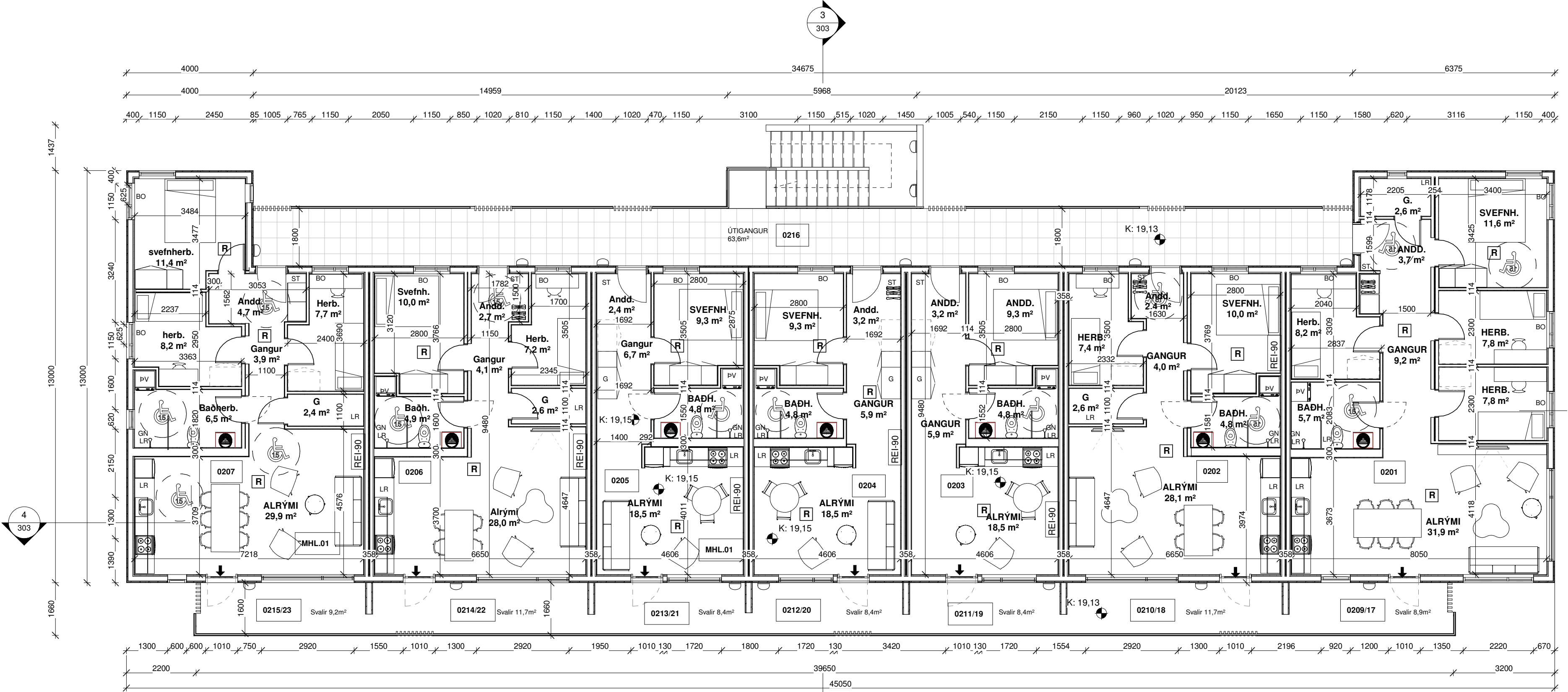
GRUNNMYND 2. HÆÐ Heiðarsteckur 1 1 : 100
