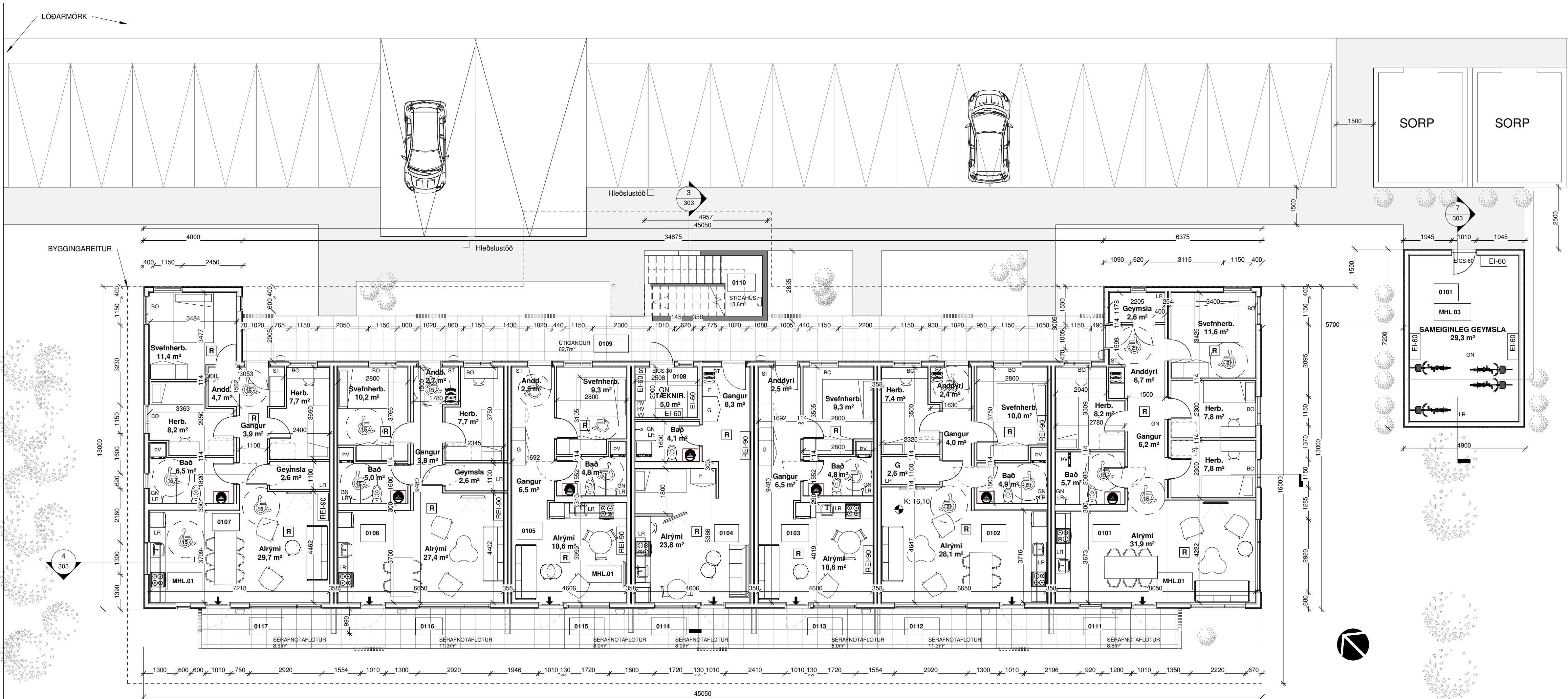
GRUNNMYND 1. HÆÐ Heiðarsteckur 1 1 : 100
