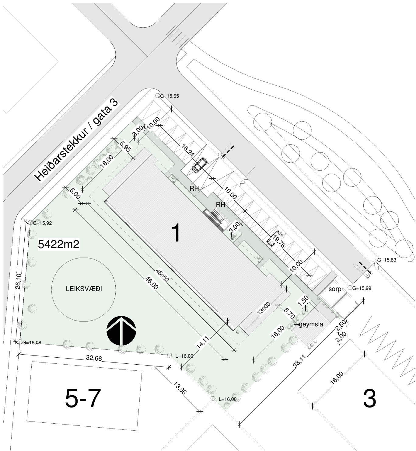
AFSTÖÐUMYND HEIÐARSTEKKUR 1 1 : 500
