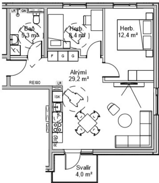
3.Herbergi_týpa A 1 : 100
