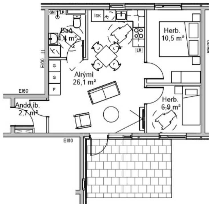
3.Herbergi_týpa B 1 : 100
