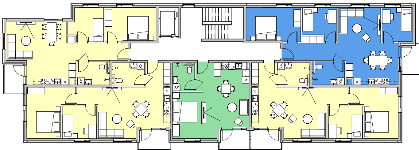
Hæð 4 1 : 200
