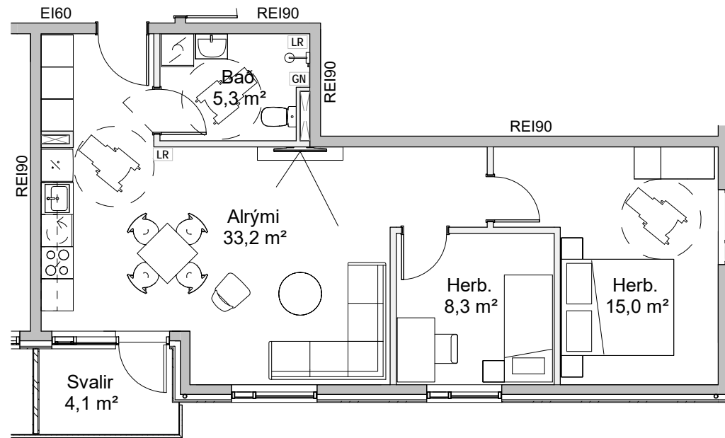
3.Herbergi_B 1 : 100
