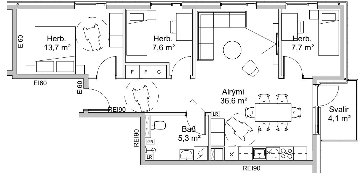
4.Herbergi 1 : 100
