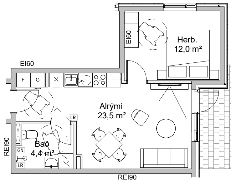
2.Herbergi_A 1 : 100
