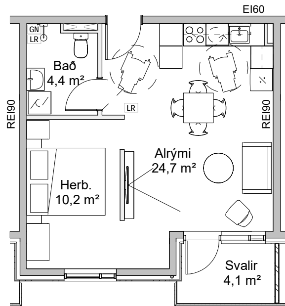
2.Herbergi_B 1 : 100
