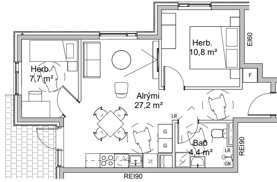
3.Herbergi_A 1 : 100
