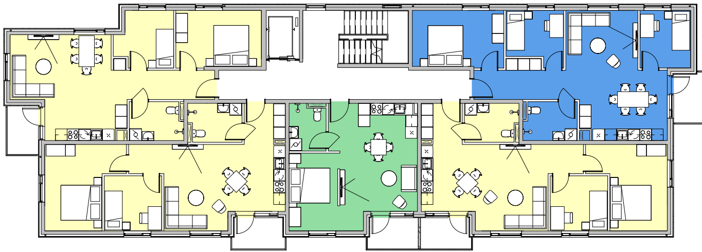
Hæð 3 1 : 200
